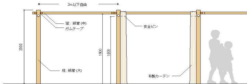
立面図 S=1/30
