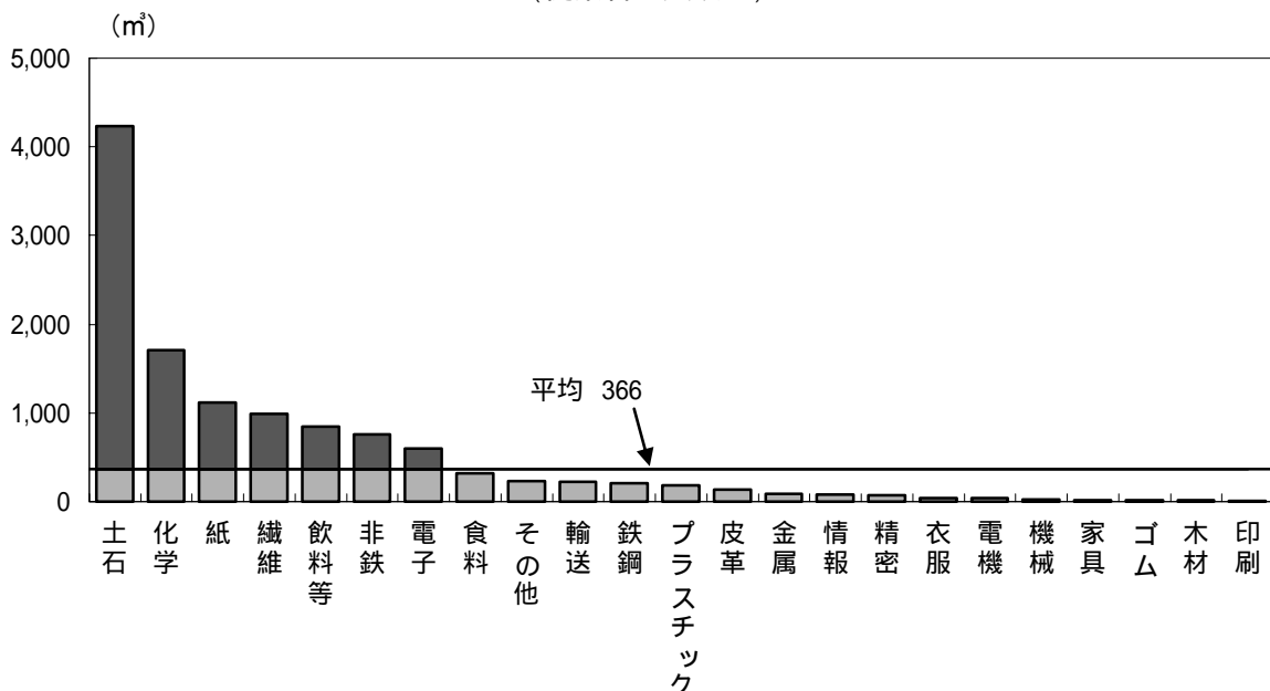
図12-4 1事業所当たり工業用水(淡水)使用量 (従業者30人以上)
