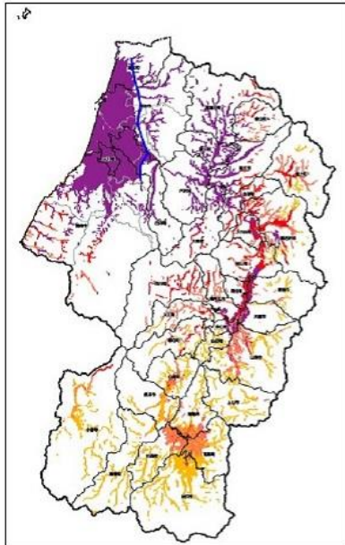
庄内平野東縁断層帯地震
