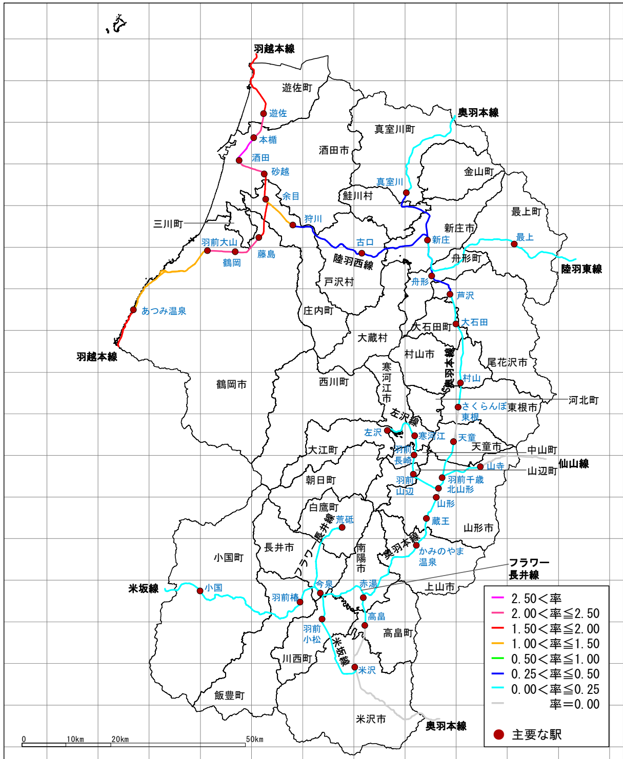
図4.2.2 鉄道施設被害率 F34断層地震
