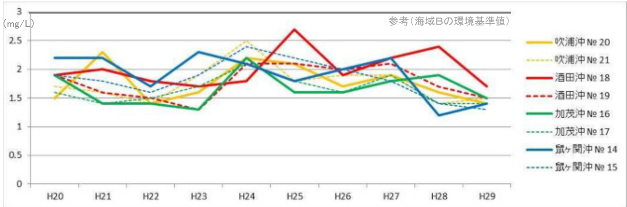
過去10年間におけるCOD75%値の状況
