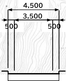
現況横断面
