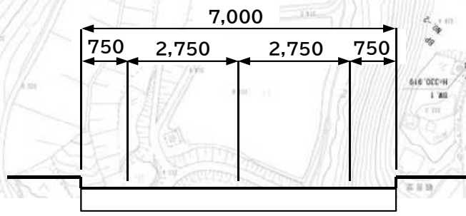
計画横断面
