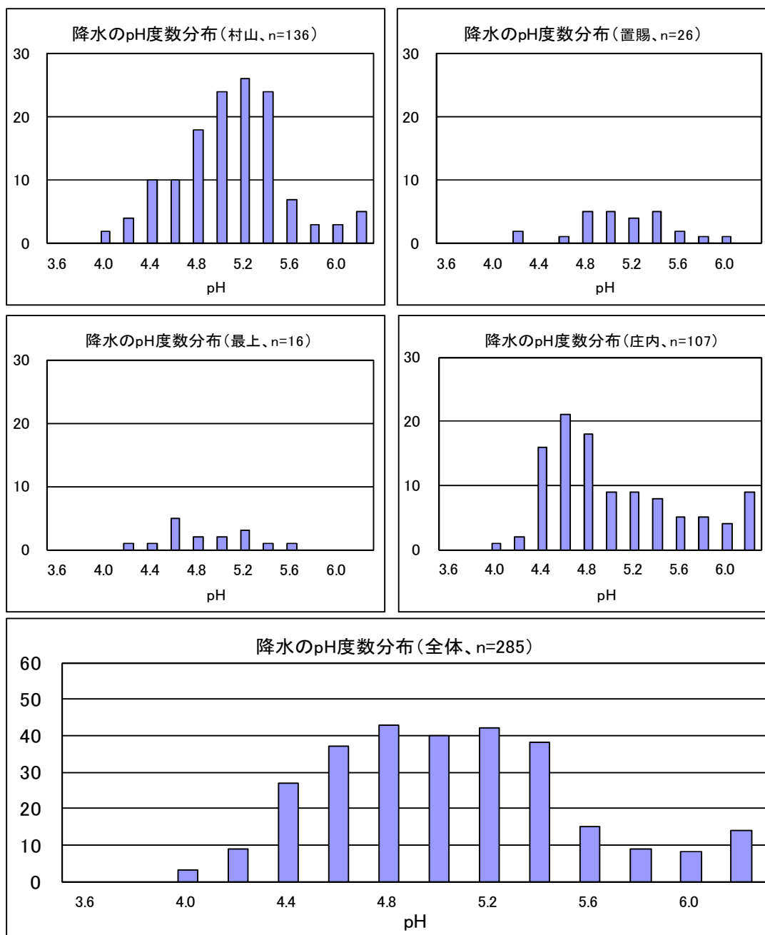
図-2 降水の pH の度数分布
