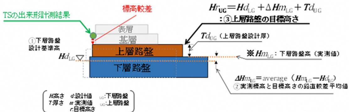
図-3 オフセット高さと標高較差
