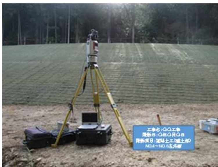
図－3 写真撮影例
