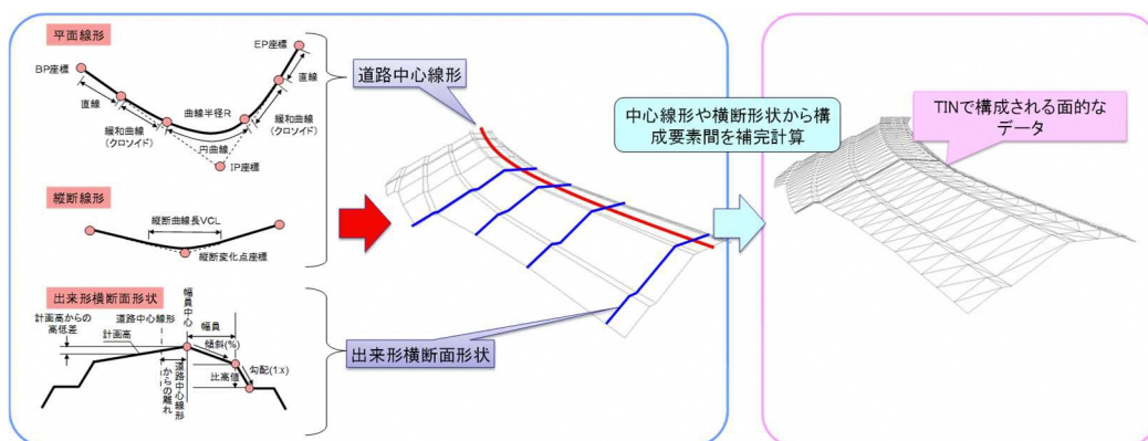
図－4 3次元設計データのイメージ（道路土工の場合）
