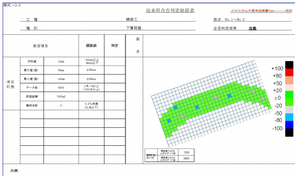
図-4. 1 作成帳票例 (出来形管理図表・標高較差)
