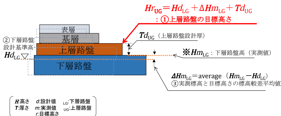
図-3 目標高さ（例：アスファルト舗装）
