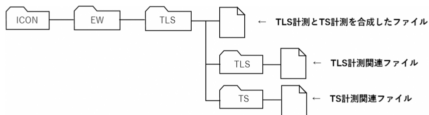
図 5-8 TLS計測を主としTSにて欠測補間した場合の構成例
