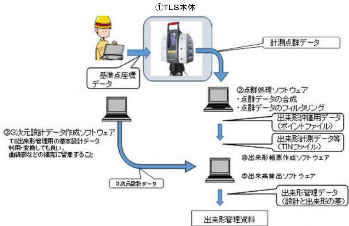
図 2-1 TLSによる出来形管理機器の構成例
