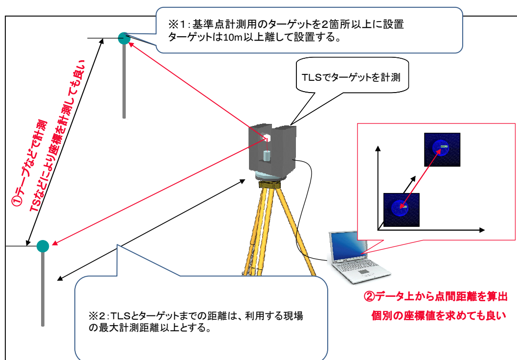
図- 4-2 TLSと既知点の設置
