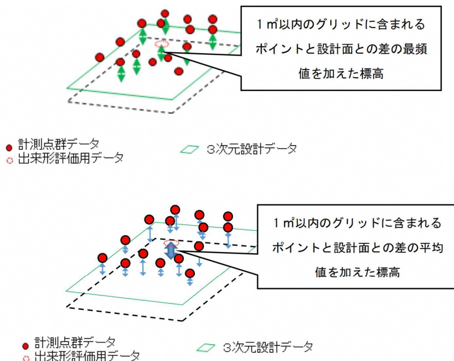
図 2-3 グリッドデータ化のイメージ
