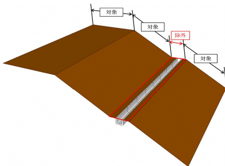
図 4-5 構造物が設置されている小段
