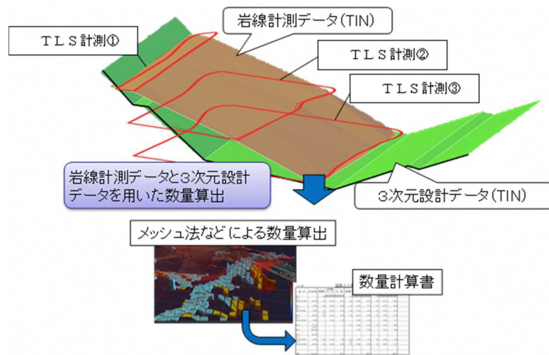
図 3-2 設計変更（岩区分）のための数量算出イメージ
