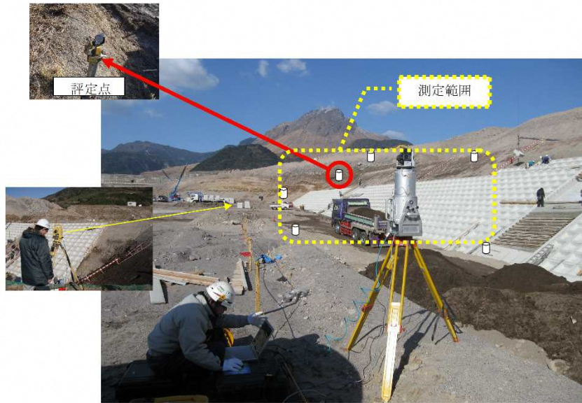
図 4-3 TLSと標定点の配置 (例)
