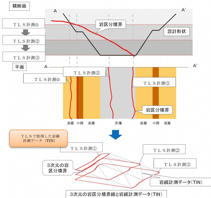
図 3-3 TLSで取得する岩区分境界のイメージ
