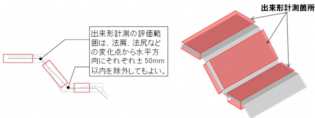
図 4-4 出来形計測箇所
