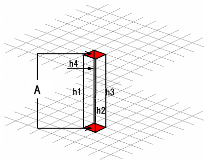
図 5-5 点高法による数量算出
