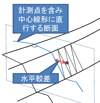
図 2-4 水平較差の算出ロジックのイメージ
