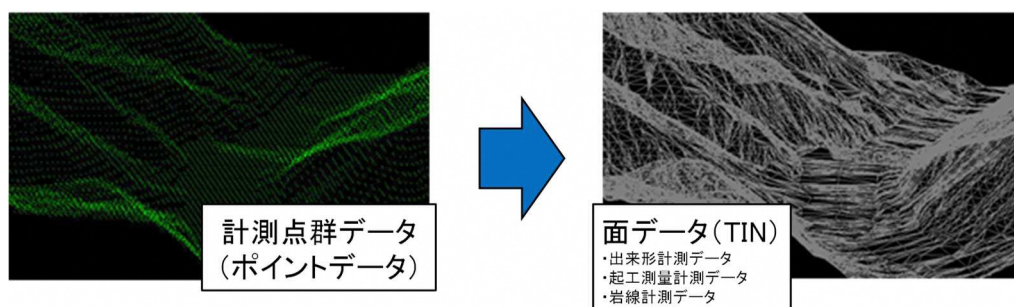
図 2-3 計測点群データをT I Nデータに変換する方法
