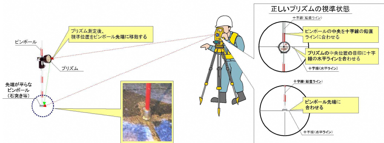
図一 1 プリズムを視準する位置
