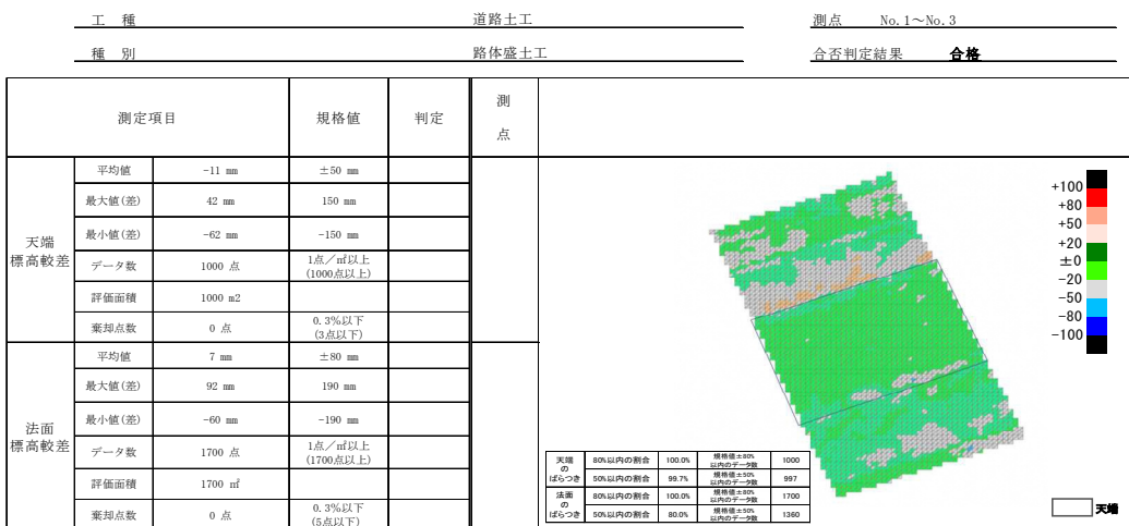
図 5-2 出来形管理図表 作成例 (合格の場合)
