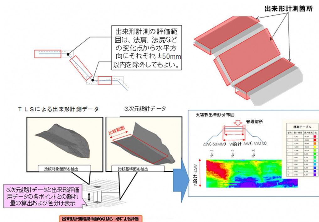
図 2-6 面的な出来形管理分布図のイメージ
