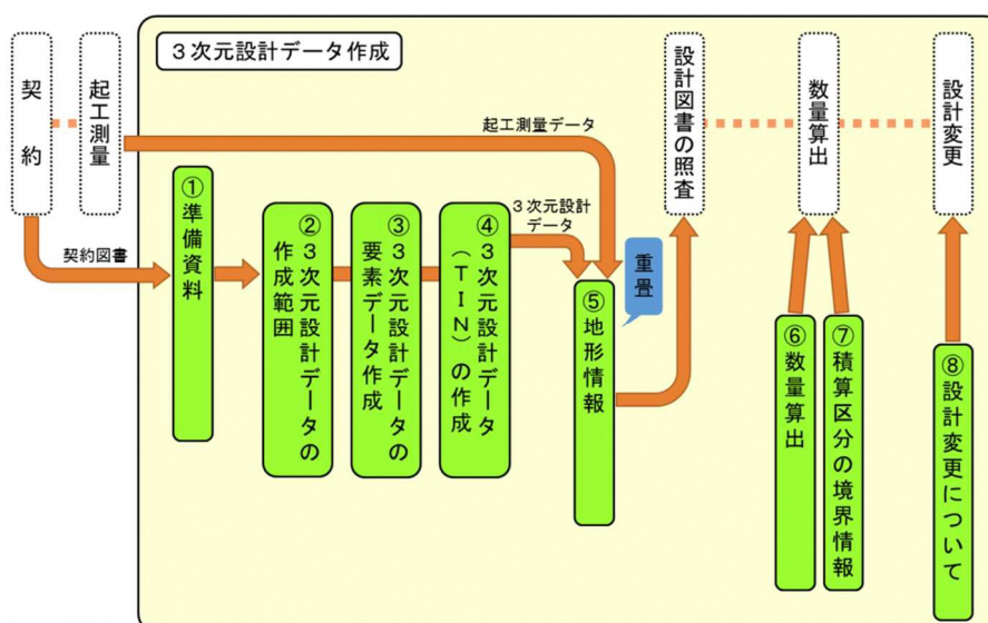
図 4-2 3次元設計データの流れ
