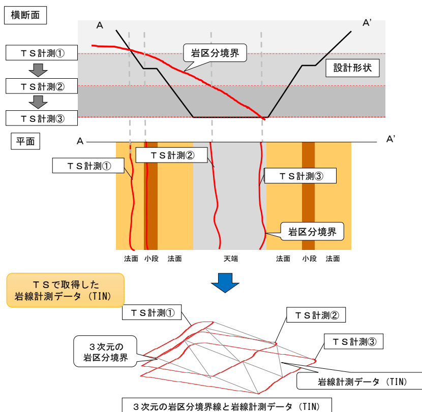
図 3-3 TS（ノンプリズム方式）で取得する岩区分境界のイメージ
