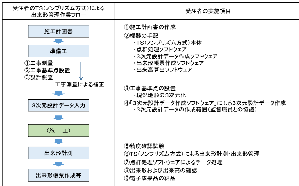
図 1-1 TS（ノンプリズム方式）による計測の手順
