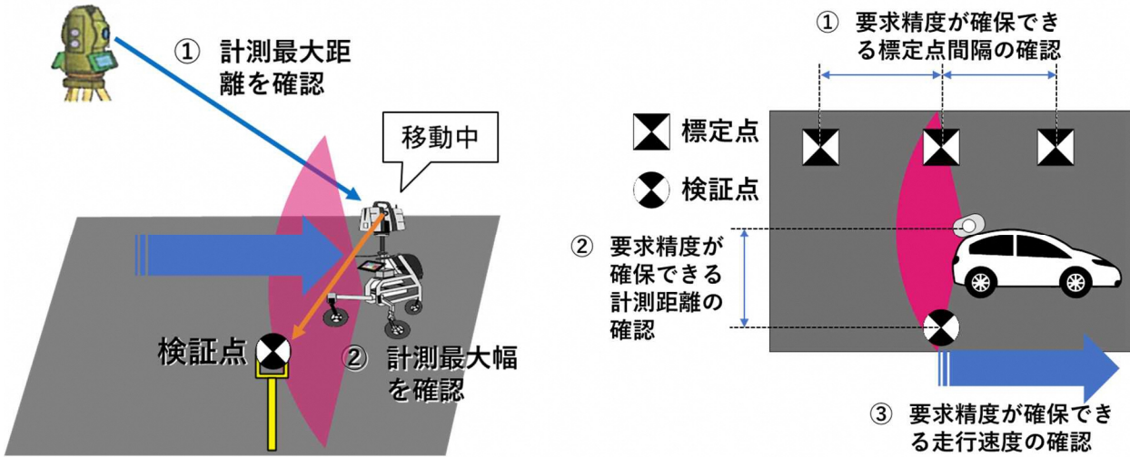
図- 4-2 精度検証の方法
