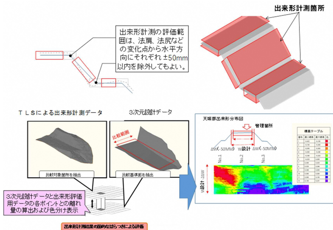
図 2-9 面的な出来形管理分布図のイメージ
