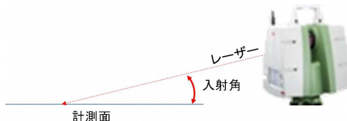
図1-3 地上移動体搭載型LSの位置と計測面との入射角
