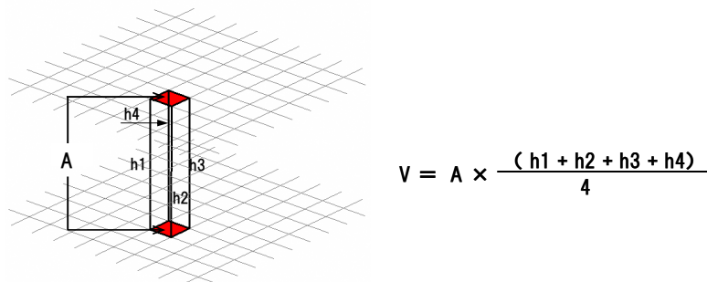
図5-5 点高法による数量算出
