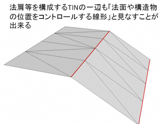
図2-8 位置をコントロールする線形
