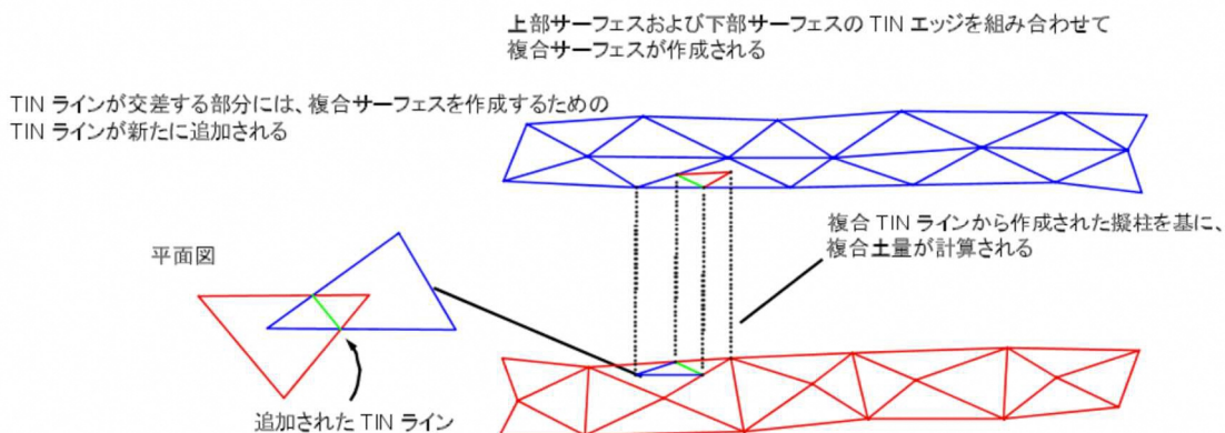
図5-7 プリズモイダル法による数量算出
