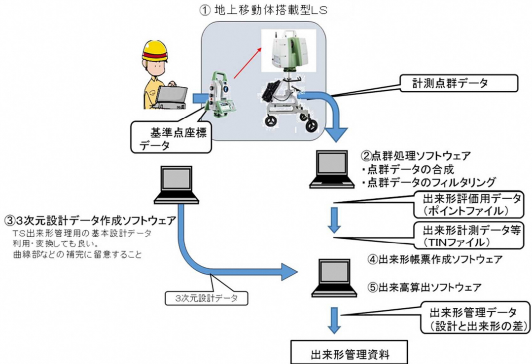
図 2 - 1 地上移動体搭載型 L S による出来形管理機器の構成例 ( 1 )
