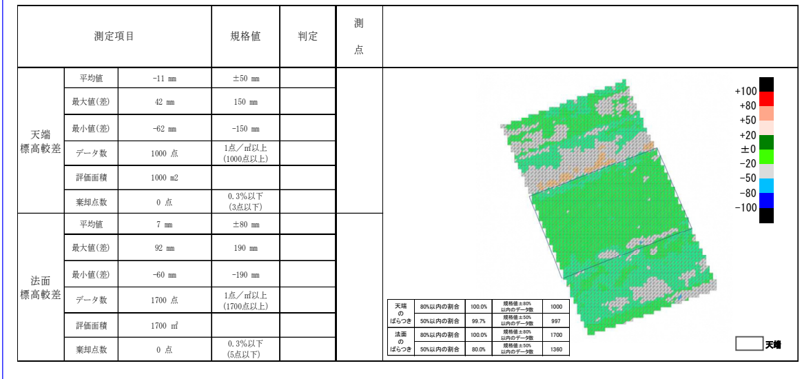
図5-2 出来形管理図表 作成例 (合格の場合)
