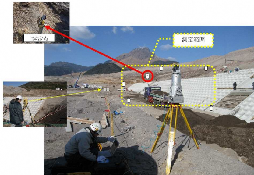
図 4-3 地上移動体搭載型 L S と標定点の配置 (例)
