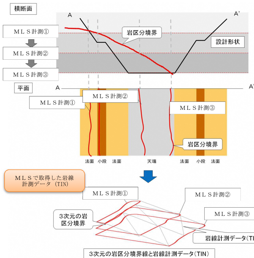
図3-3 地上移動体搭載型LSで取得する岩区分境界のイメージ
