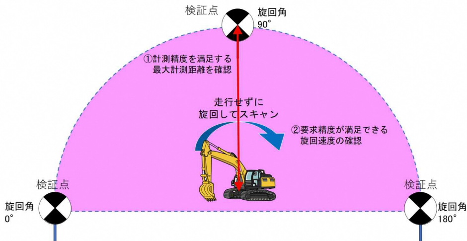
図- 4-2 精度検証の方法
