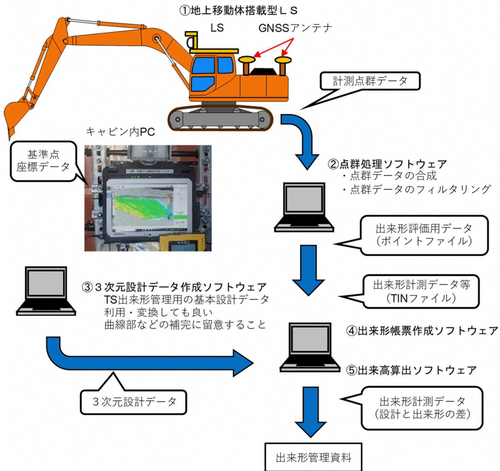
図 2 - 1 地上移動体搭載型 L S による出来形管理機器の構成例 ( 2 )
