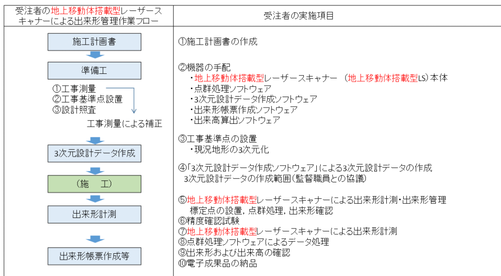
図1-1 出来形管理の主な手順
