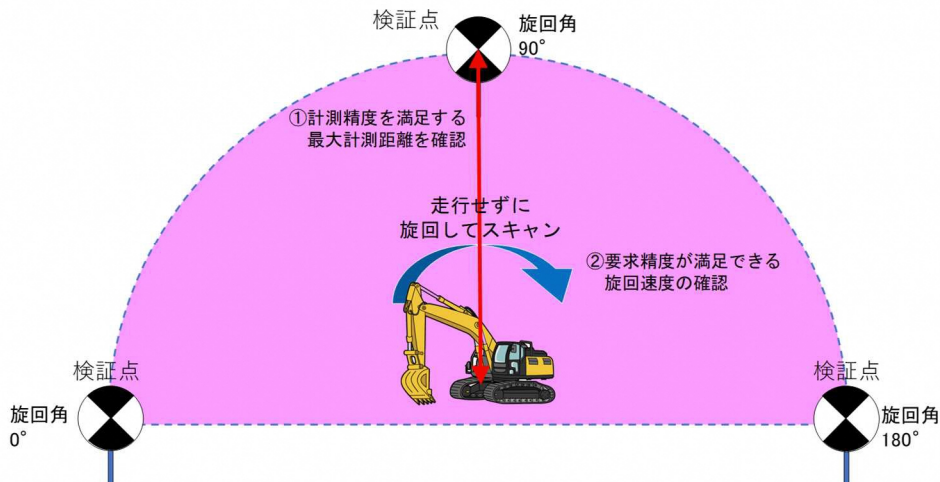
図-4-1 精度確認試験の配置イメージ図
