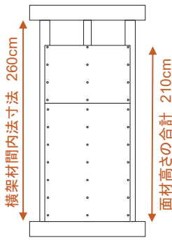
面材(構造用合板)の場合
