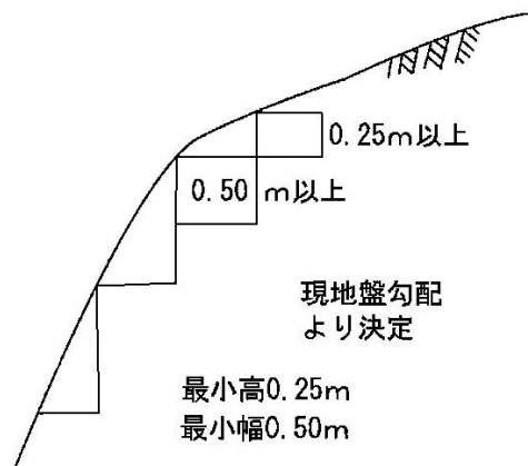
現地盤が岩の場合
