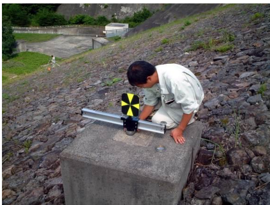
◆前川ダム 堤体移動量測量
