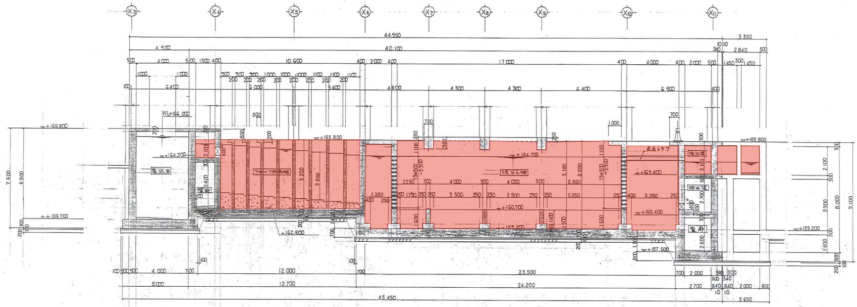
A-A 断面図 1/100
