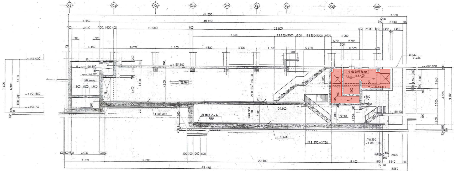
B-B 断面図 1/100
