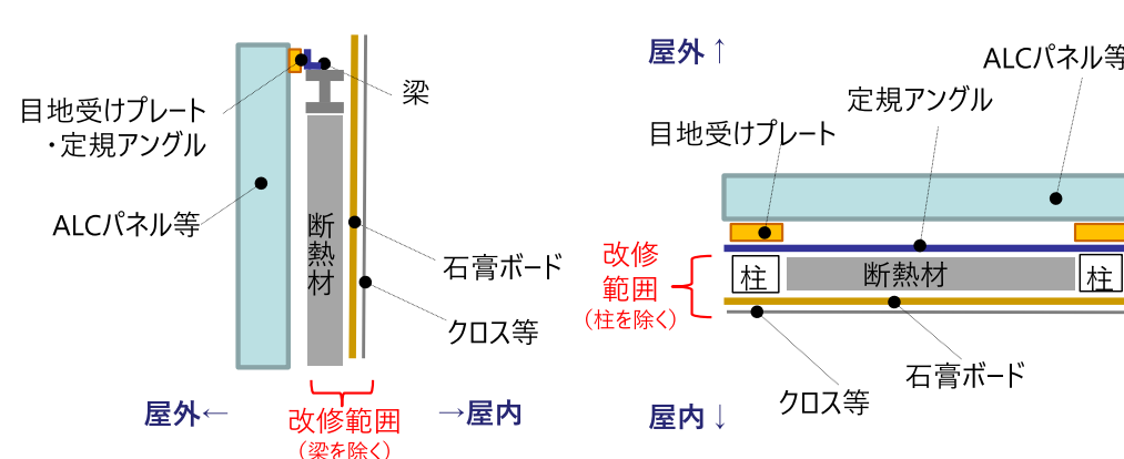
図2-3 横から見た断面図
