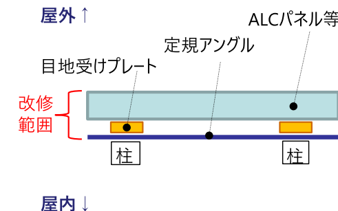
図2-8 上から見た断面図
