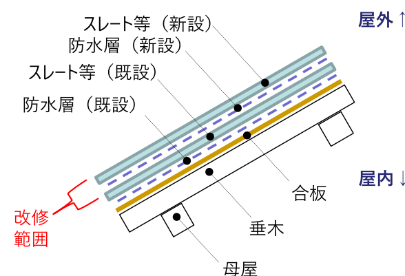
図2 横から見た断面図
