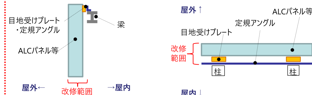
図2-7 横から見た断面図
