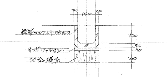
③ U形側溝 1/20
