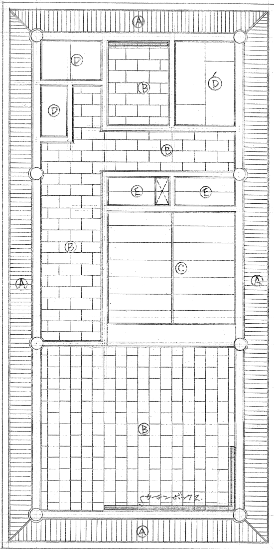
天井伏也図
