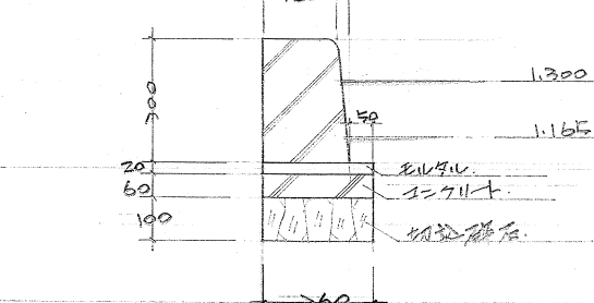
④ 縁石 1/20
