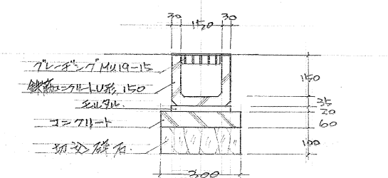
② グレーティング付U形側溝 1/20
