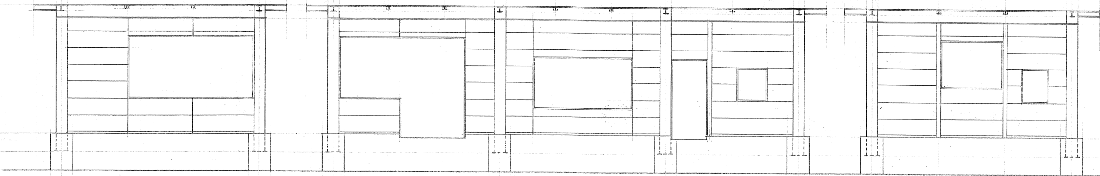
南面軸組図
