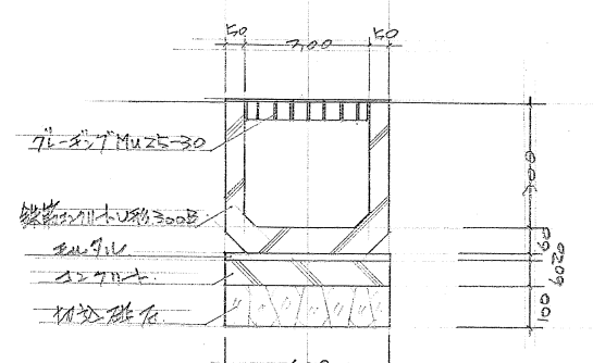
① グレーティング付U形側溝 1/20
