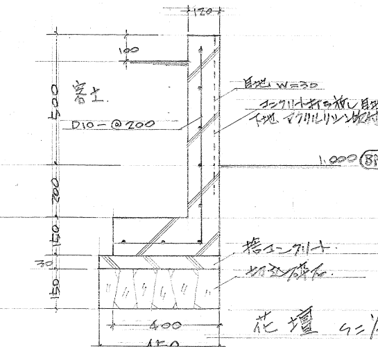
⑥ 花壇 1/20
