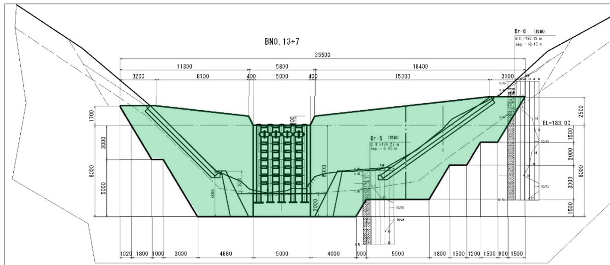
〔砂防えん堤正面図〕
