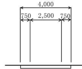
現況横断面図
