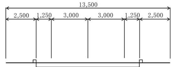
計画横断面図
