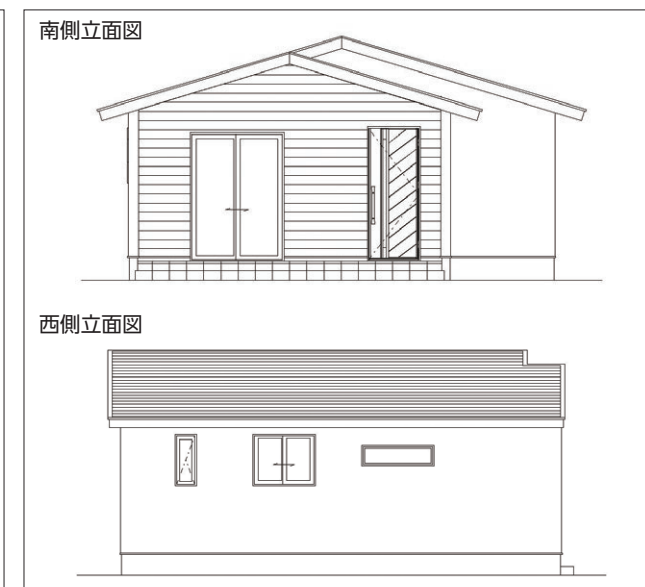
立面図2面
