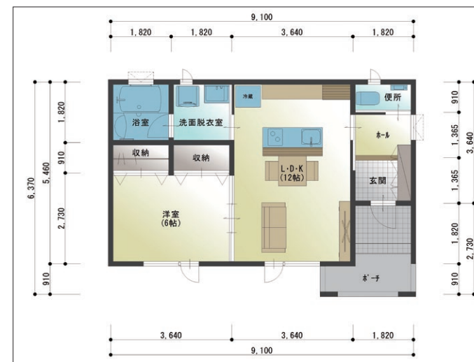
一階平面図
