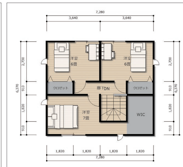
二階平面図
