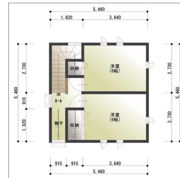
二階平面図
