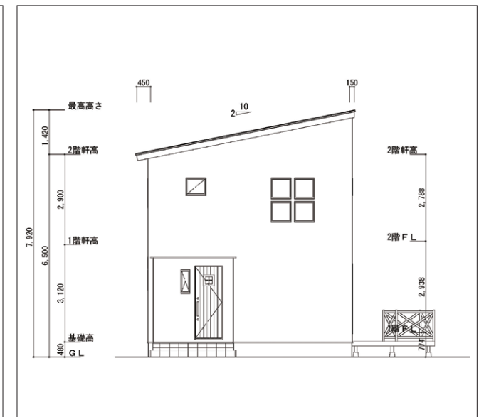
立面図
