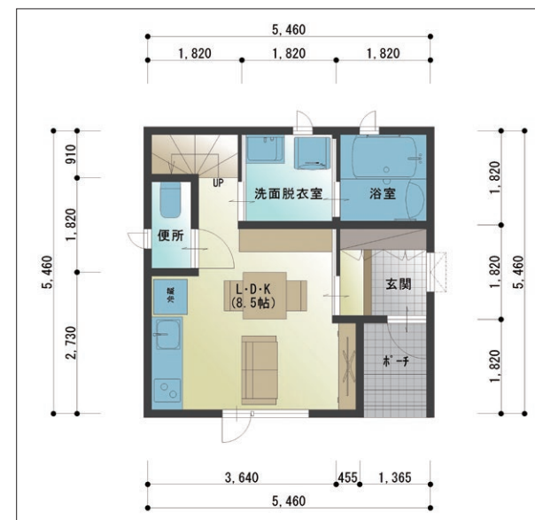
一階平面図
