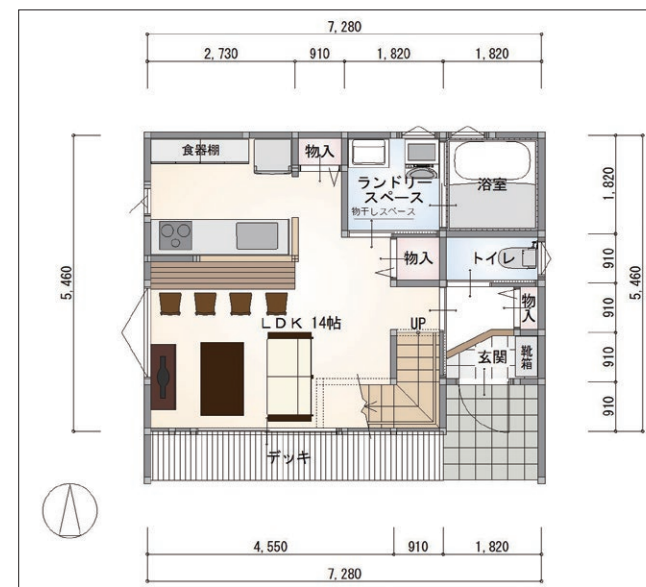
一階平面図
