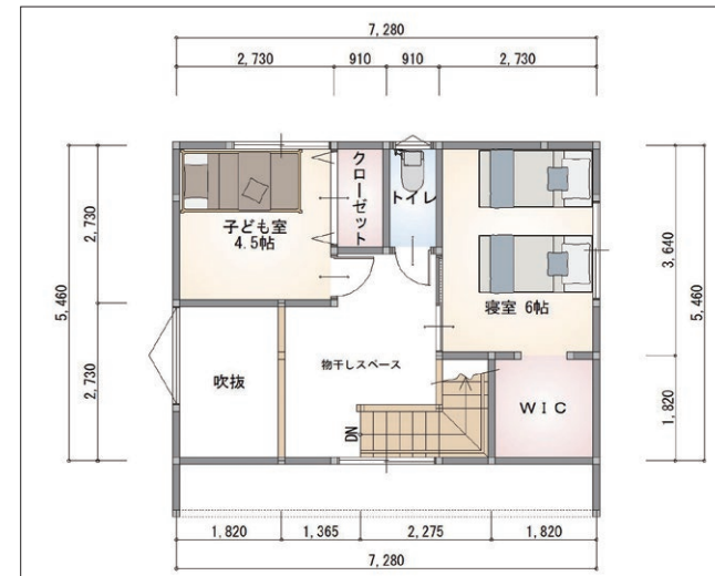
二階平面図
