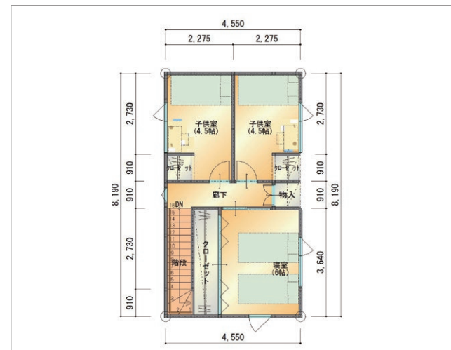
二階平面図
