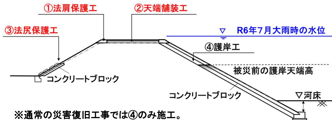
【横断模式図】
