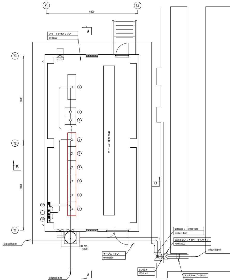
沈澱池電気室配置 平面図
