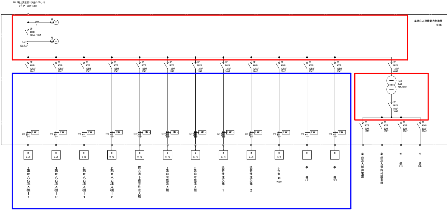
薬品注入設備動力制御盤単線結線図
