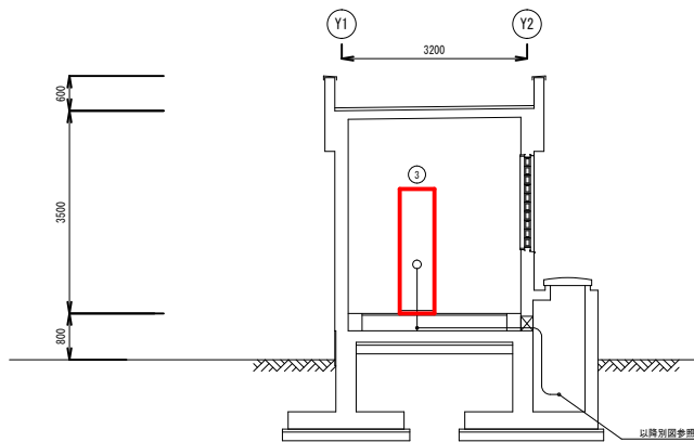
A-A断面図 5:1 : 50
