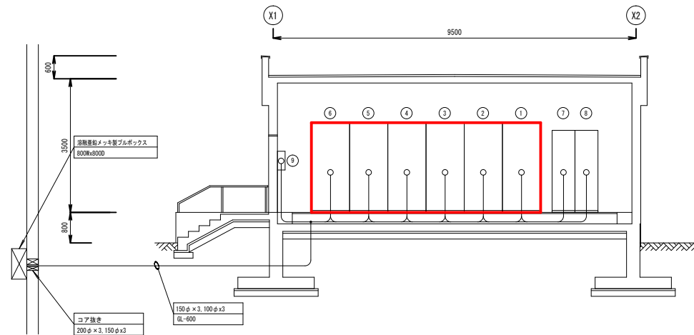
B-B断面図 5:1 : 50
