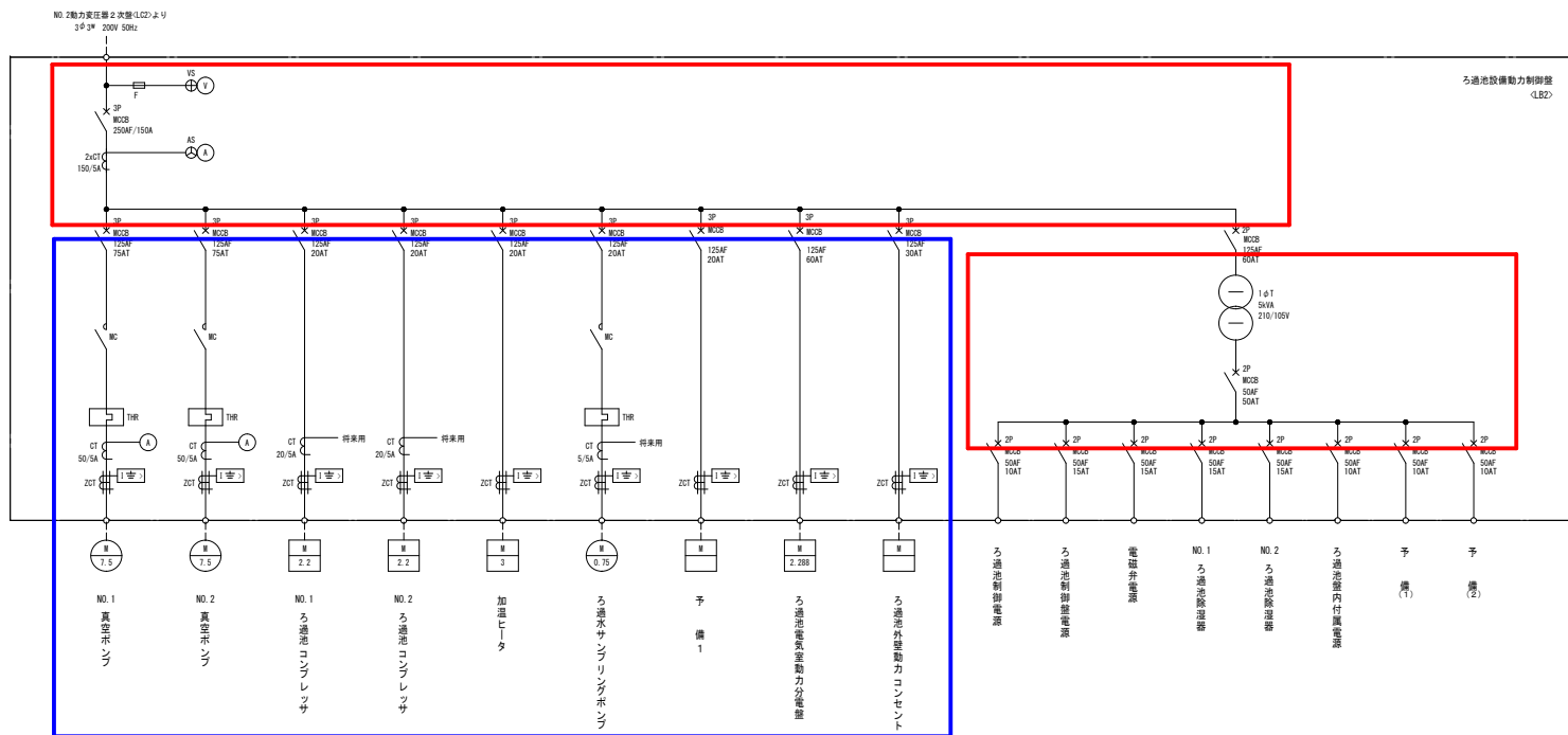
ろ過池設備動力制御盤単線結線図
