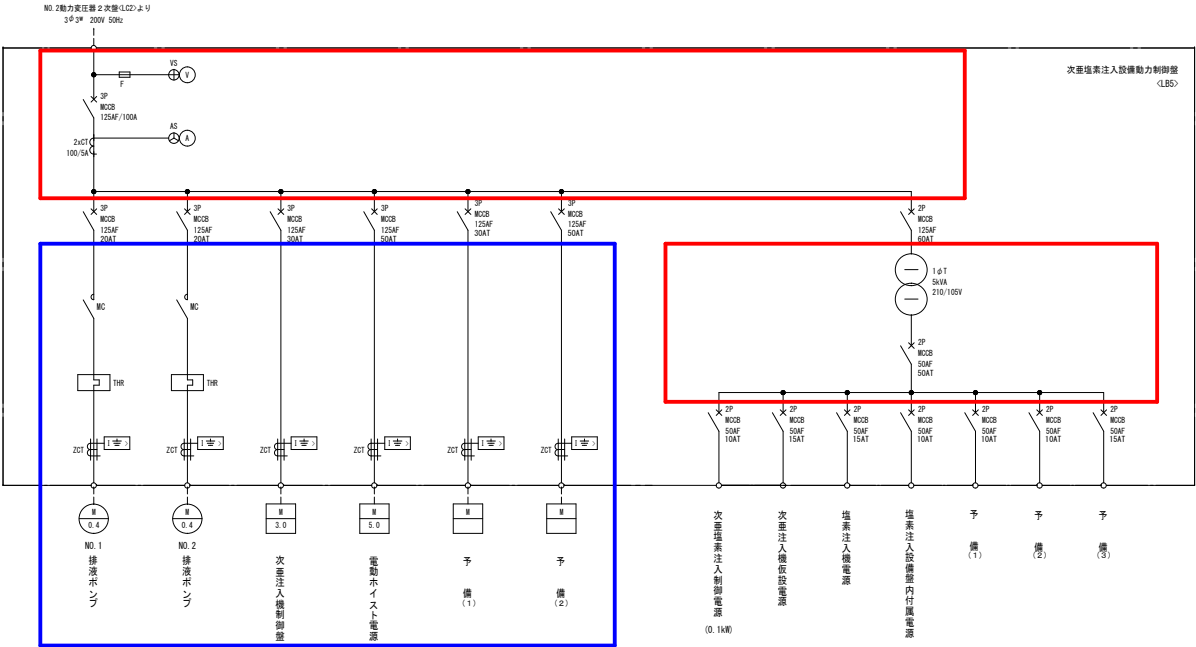
次亜塩素注入設備動力制御盤単線結線図
