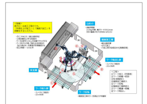
支援報告書例 装置の構想図
